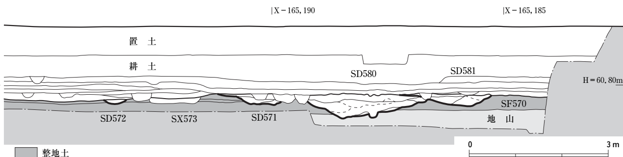
図84 西壁断面図 1:80
