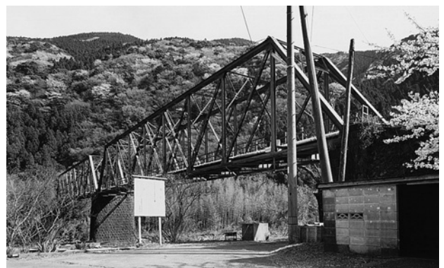
図60 小島影橋 トラス橋
