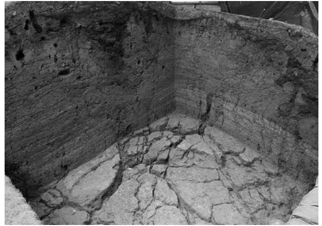
図141 版築層の断面と縦横に走る地震痕跡
