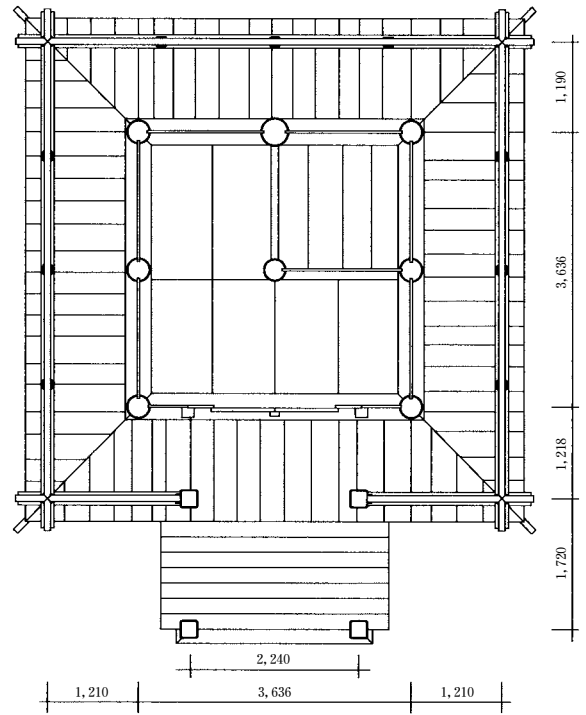
図76 命主社平面図 1 : 100
