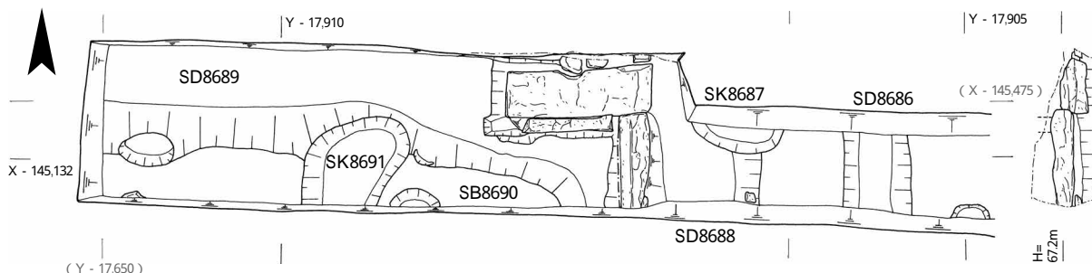
図190 光月亭南調査区遺構平面図 1 : 50
