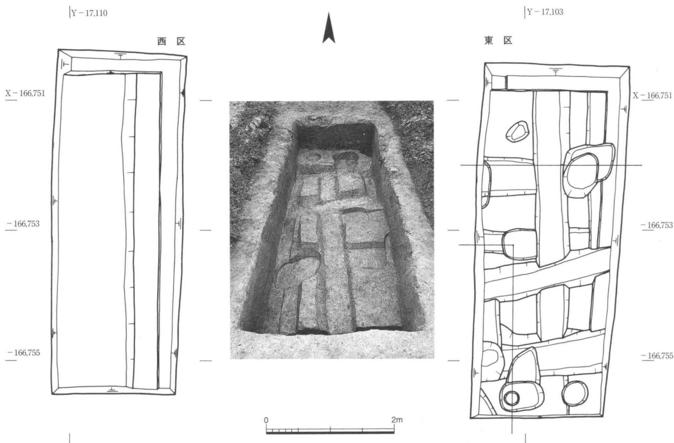
図74 第114-10次調査遺構図 1:60 写真は東区(北から)
