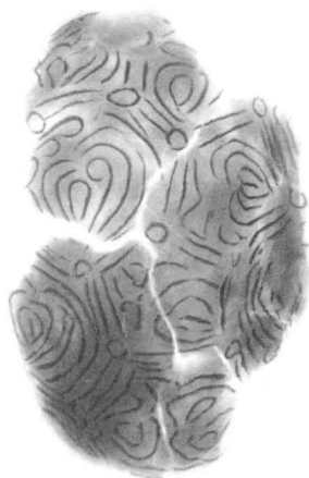
図71 島根県妙蓮寺山古墳出土太刀鉄地銀象嵌柄頭（島根県立博物館蔵）のX線ラジオグラフ 【インスタントシートフィルムを用いて得られたポジ画像】
