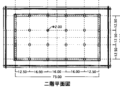
図22 平成13(2001)復原案
