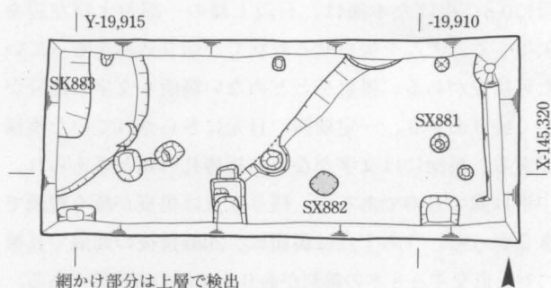
図152 第335次調査遺構平面図 1:100
