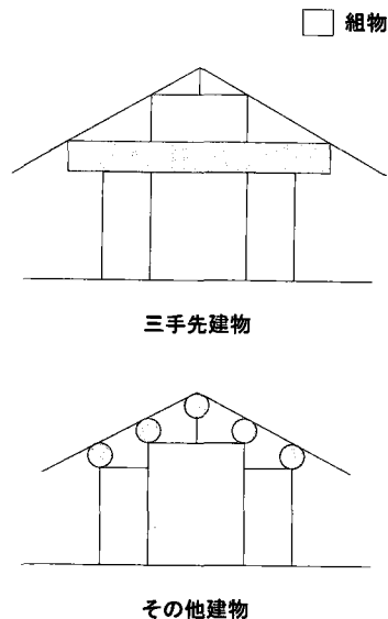
図3 三手先建物とその他建物の構造の違い
