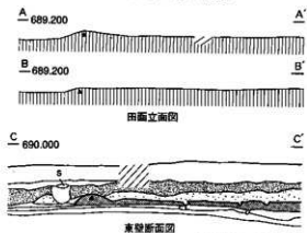
東壁断面図
