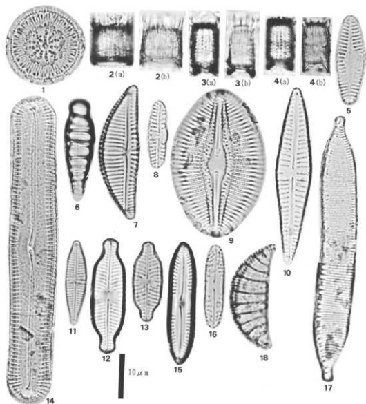
图版 1 珪藻化石
