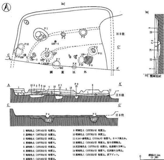
第138図 H 4 号住居址実測図
