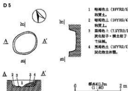
第165図 D 1～D 5号土坑址実測図 (1)
