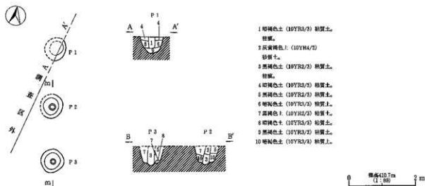
第230図 F4号掘立柱建物址実測図
