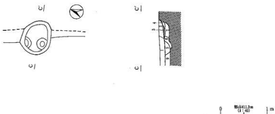
第136図 H3号住居址カマド覆り方実測図
