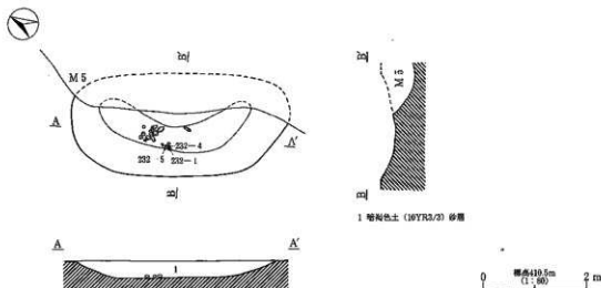
第231図 D12号土坑址実測図
