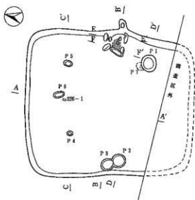
第149図 H 8号住居址実測図
