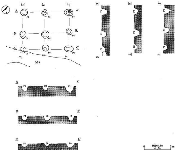
第164図 F3号掘立柱建物址実測図
