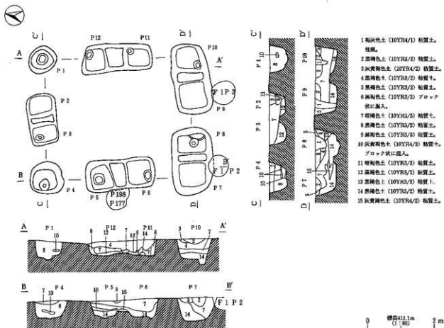
第163図 F2号掘立柱建物址実測図
