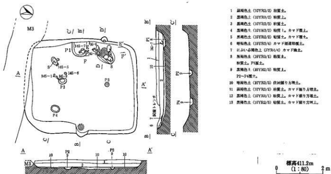
第143図 H6号住居址実測図
