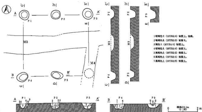
第162図 F1号掘立柱建物址実測図
