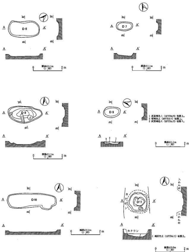
第166図 D6～D11号土坑址出実測図(2)
