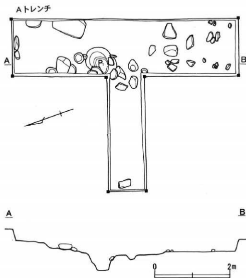
図11 Ⅲ区Aトレンチ平面図(1:50)
