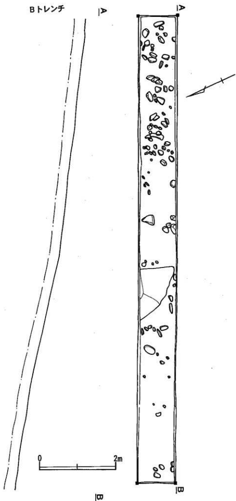
図12 III区Bトレンチ平面図 (1:50)
