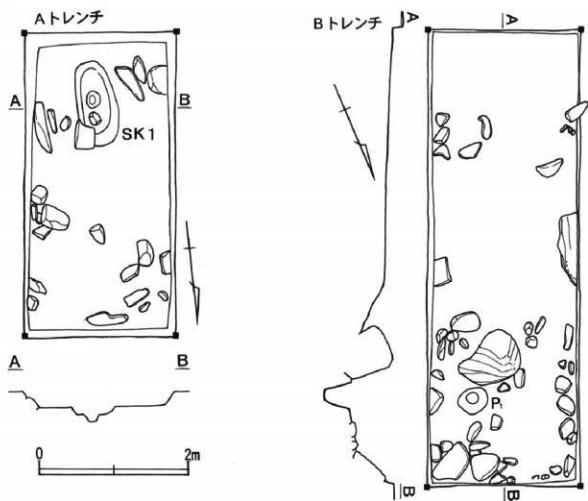
図9 I区A・Bトレンチ平面図(1:50)
