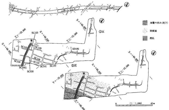
第82図 B2地区第7水田全体図
