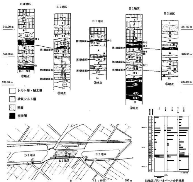
第144図 E1地区基本層序
