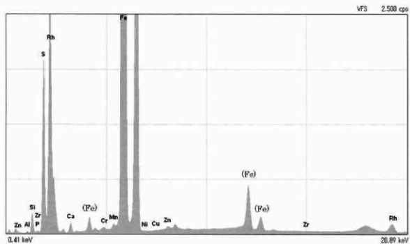
図版2. 礫裏面の鉄Feマッピング測定結果 (スペクトル図は、範囲bのマッピングによる)
