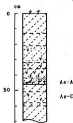
図5 D地点の土層柱状図
