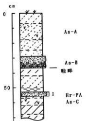
図4 C地点の土層柱状図 数字はテフラ分析番号
