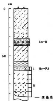
図7 G地点の土層柱状図
