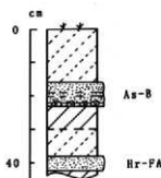
図6 E地点の土層柱状図
