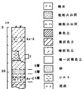
図2 A-2地点の土層柱状図 数字はテフラ分析番号
