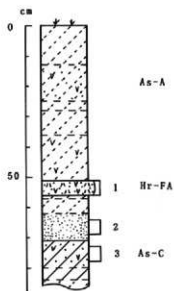
図3 B地点の土層柱状図 数字はテフラ分析番号
