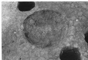
3-1-3号土坑全景 (南より) 04-00019-06
