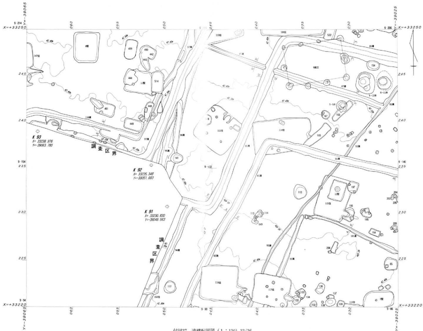
付図37 遺構配置図 (1 : 120) 33/36
