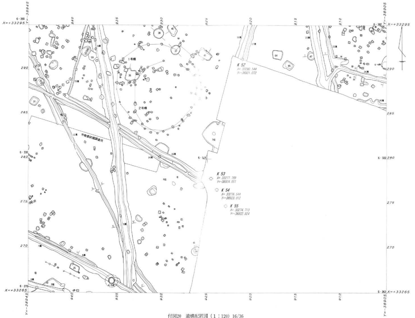
付図20 遺構配置図 (1:120) 16/36
