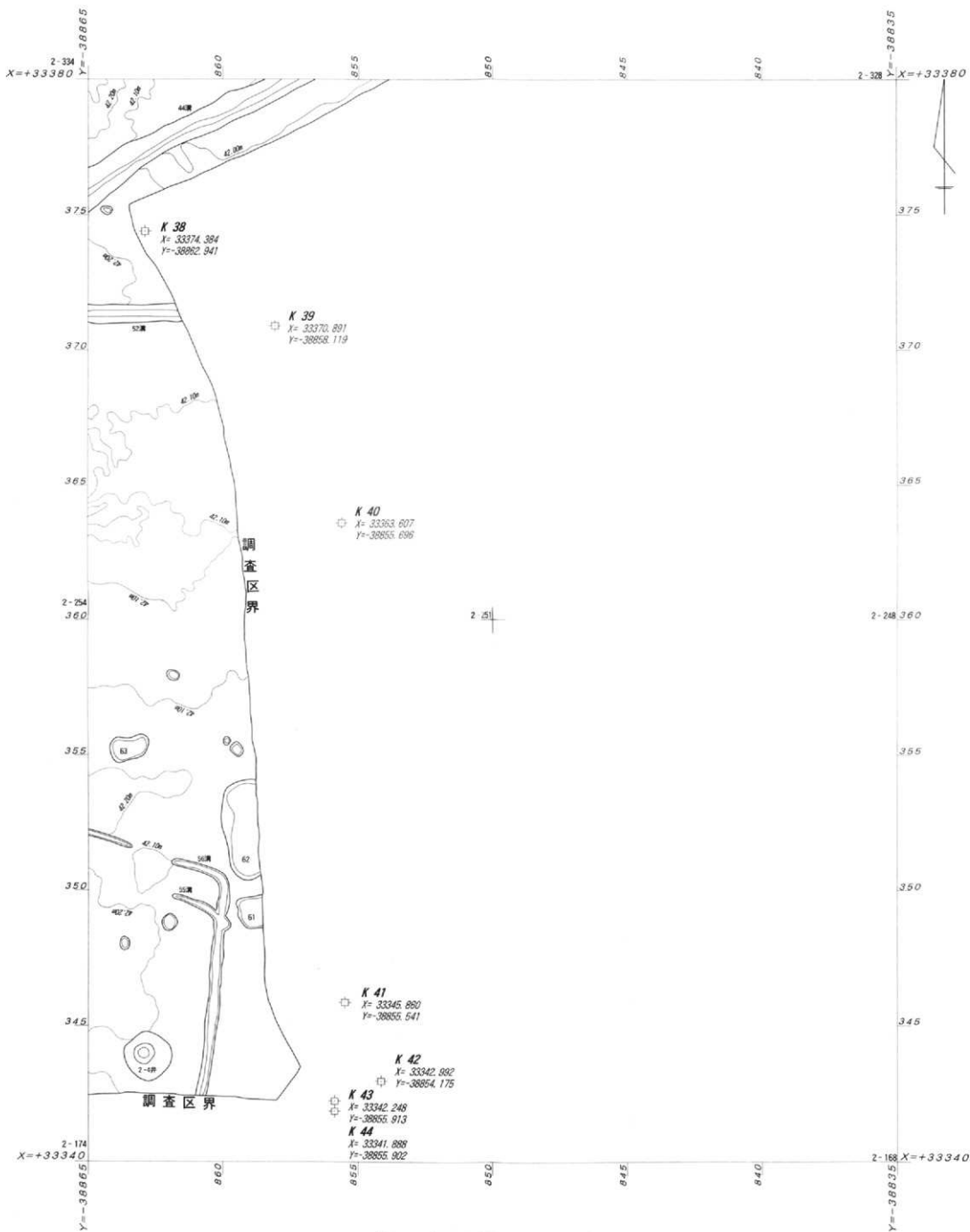
付図6 遺構配置図 (1:120) 2/36
