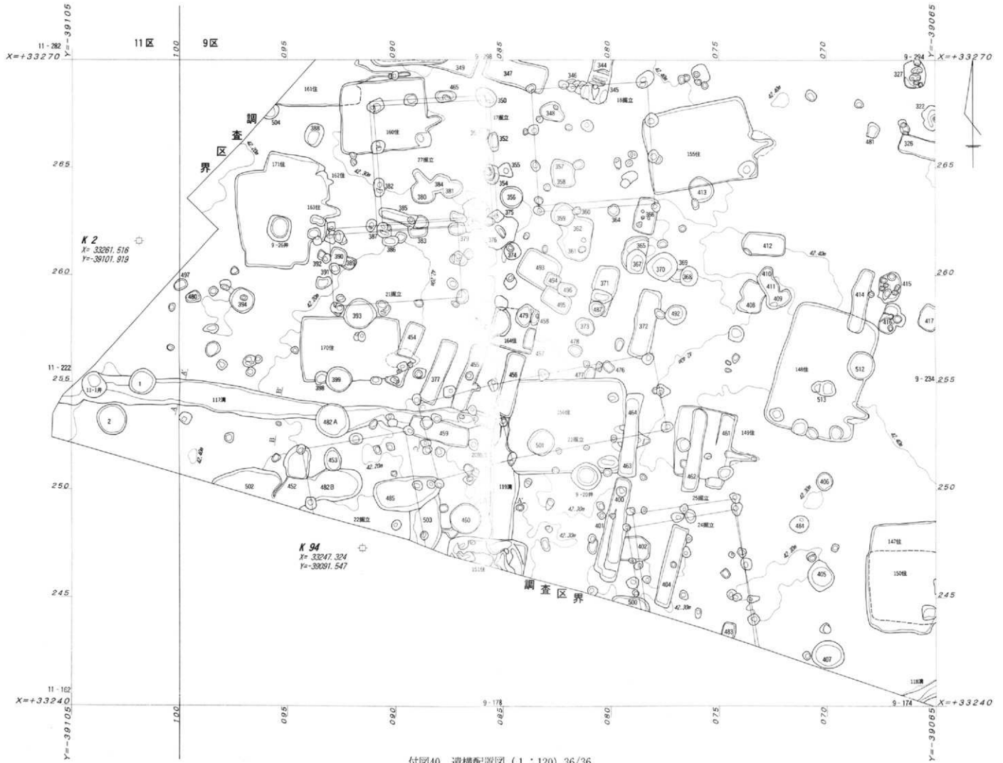
付図40 遺構配置図 (1:120) 36/36
