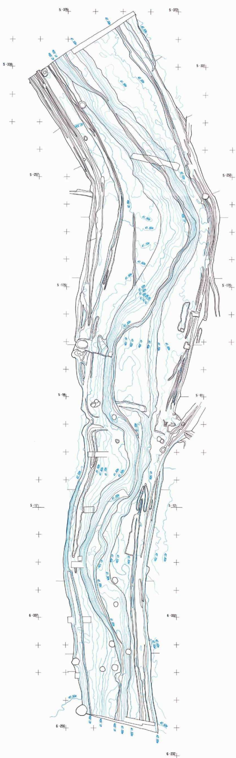
付图3 第1号坝第2·3面平面图(1:200)
