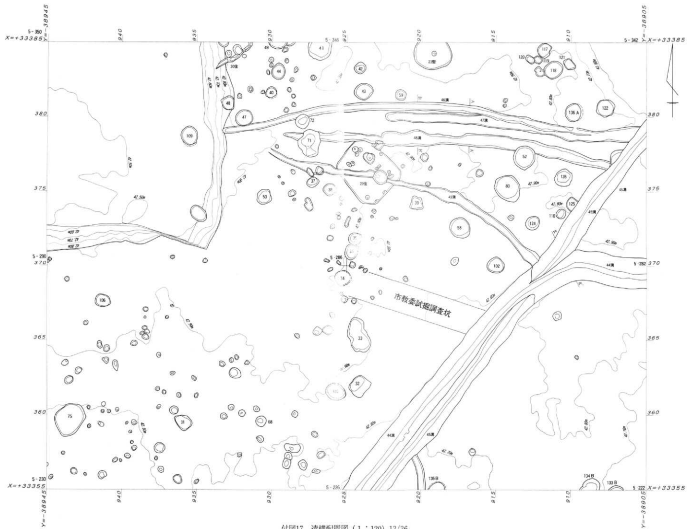
付圖17 遺構配置圖 (1:120) 13/36
