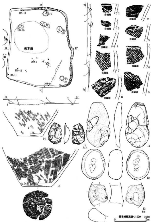
第109圖 第32号住居跡・出土遺物実測圖
