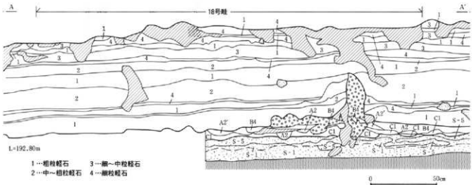
第89図 18号畦断面図
