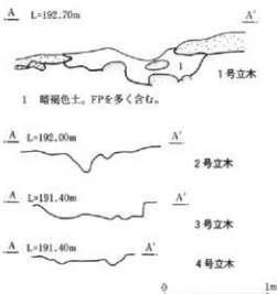
第122図 1号・2号・3号・4号立木断面図
