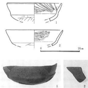
第65図 4-Aブロック出土遺物
