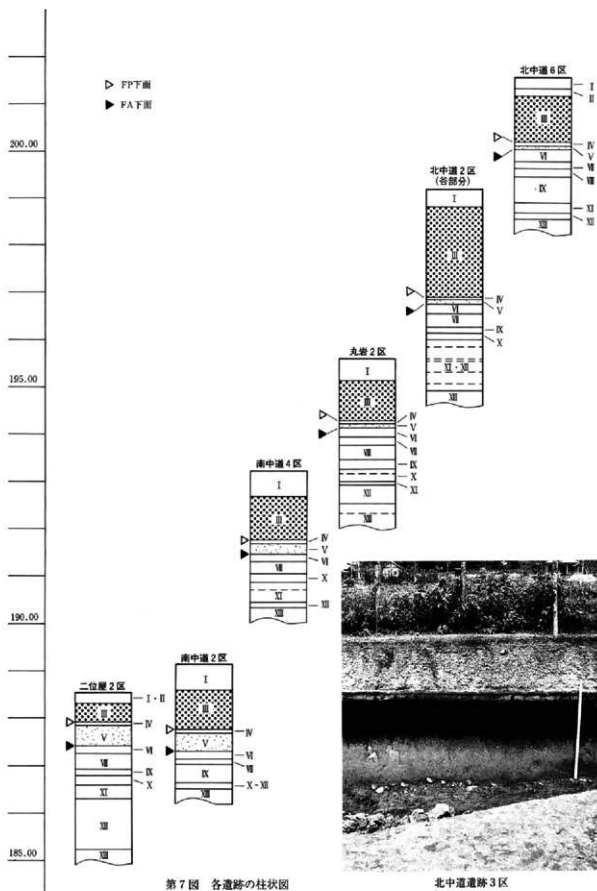
第7図 各遺跡の柱状図
