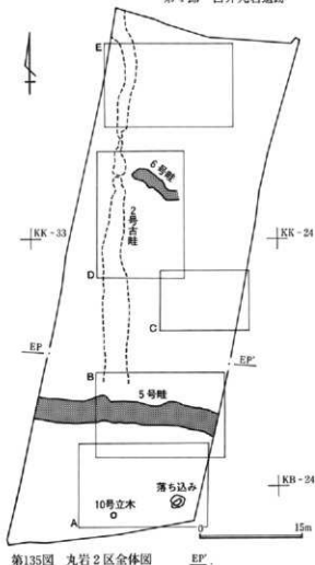
第135図 丸岩2区全体図
