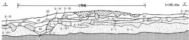
第28図 12号畦断面図
