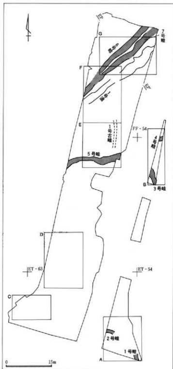
第31図 南中道2区全体図
