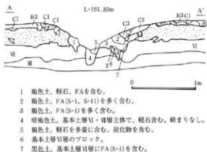
第87図 14号立木断面図
