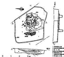
原山B遺跡1号竪穴実測図
