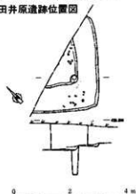
3号住居跡実測図
