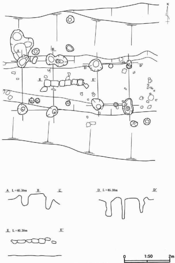
第171図 3号溝木橋柱跡
