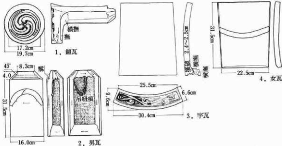
第311図 宮下西遺跡出土中世瓦復原図
