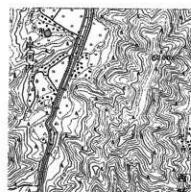
遺跡の位置(1/25000「上直見」)
