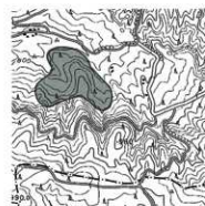
No.18 尾ノ嶽遺跡 (S=1/25000「立門」)
