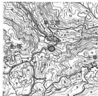
遺跡位置図（1/25000「天ヶ瀬」）
