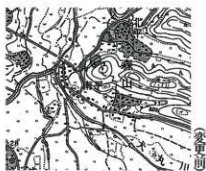
No.17 洗添横穴墓群 (S=1/25000 「土佐井」)
