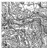
遺跡位置図 (1/25000「日田」)
