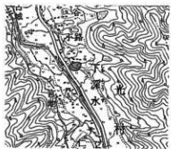
No.8 下深水小路遺跡群 (S=1/25000「宇佐」)
