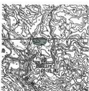
No.5 小園久保遺跡 (S=1/25000 「久住町」「桜町」)
