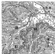
遺跡の位置(1/25000「三川内」)
