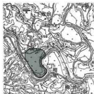
No.9 下坂田西遺跡 (S=1/25000「桜町」)
