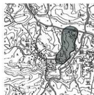
No.15 新井川遺跡 (S=1/25000「杖立」)
