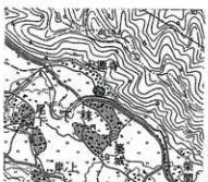
No.9 大源寺横穴墓群 (S=1/25000「土佐井」)
