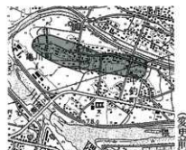
No.3 徳瀬遺跡 (S=1/25000「日田」)
