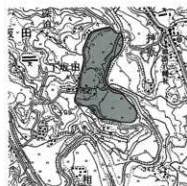
No.10 下坂田東遺跡 (S=1/25000「桜町」)
