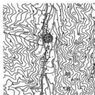
No.8 諸田山神社遺跡 (S=1/25000「両子山」)
