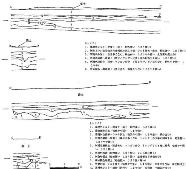
第12図 2002-05地点 トレンチ断面図(上:トレンチ1、下:トレンチ2)
