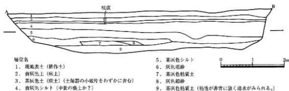
第8図 2002-06 地点 北壁断面図
