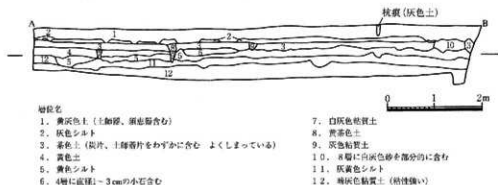
第23図 2002-10地点 南壁断面図
