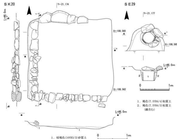
第14図 北地区遺構実測図(4)
