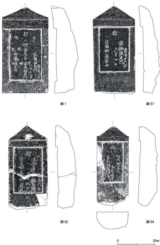
第148図 石造物実測図(3)
