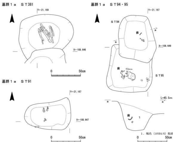
第71図 墓群1 ST 381・91・94・95実測図
