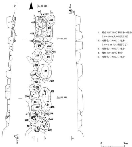
第106図 墓群16 平面・断面図
