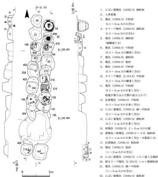
第92図 墓群12 平面・断面図
