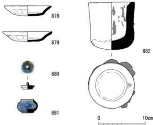
第126図 南地区墓地出土遺物実測図(9)
