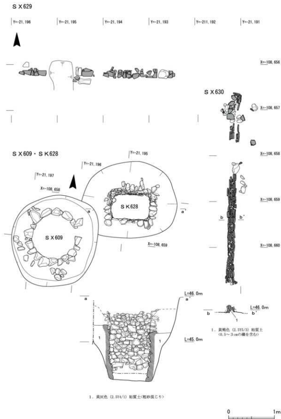
第46図 南地区遺構実測図(8)
