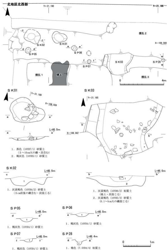
第11図 北地区遺構実測図(1)
