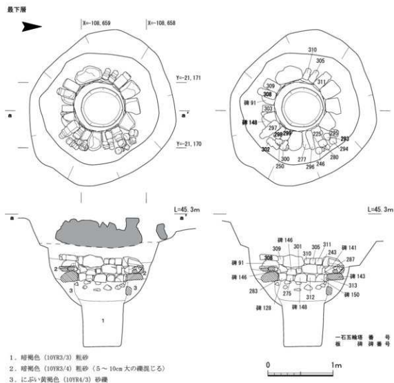
第115図 南地区SE113実測図(2)
