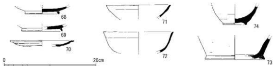
第24図 北地区出土遺物実測図(4)
