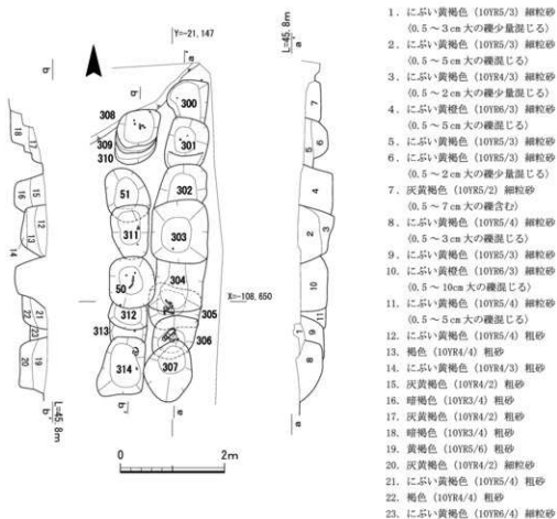
第88図 墓群10 平面・断面図
