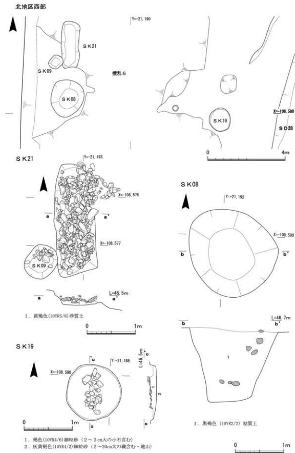
第13図 北地区遺構実測図(3)
