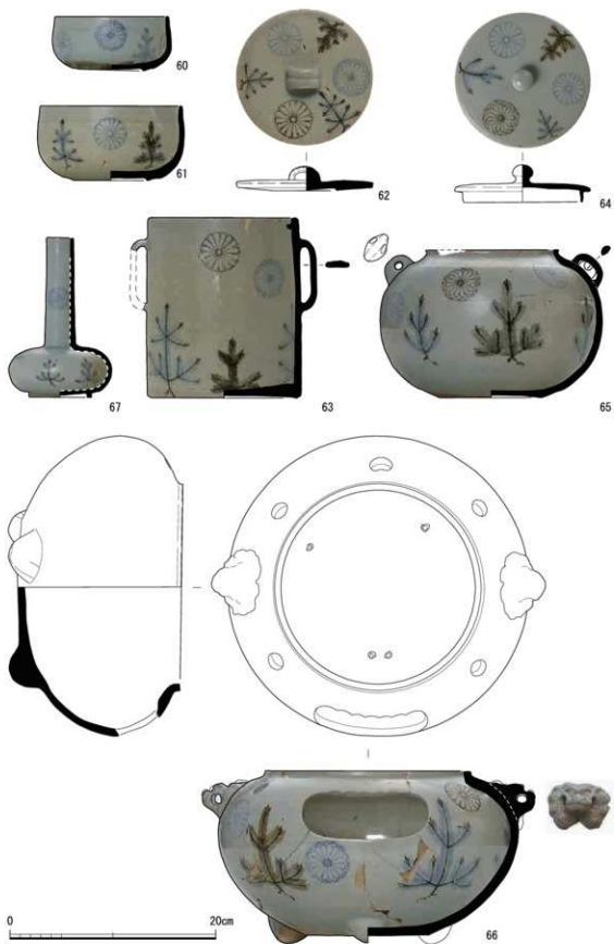
第23図 北地区出土遺物実測図(3)
