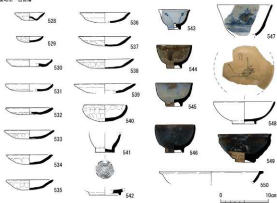
第61図 南地区出土土遺物実測図(14)
