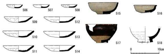
第60図 南地区出土遺物実測図(13)
