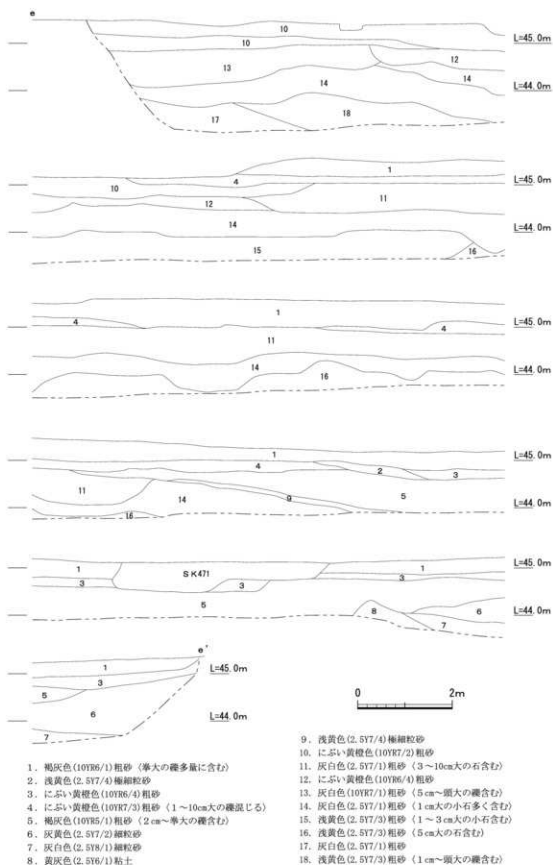
第34図 南地区土層断面図(5)
