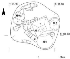
第73図 墓群2 ST21・85・67・SK66実測図
