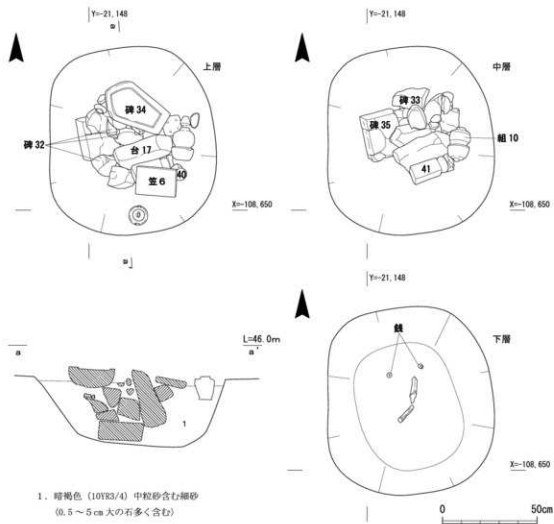
第89図 墓群10 S T50実測図
