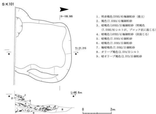
第20図 北地区遺構実測図(10)
