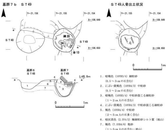
第83図 墓群6・7 S T 48・49実測図
