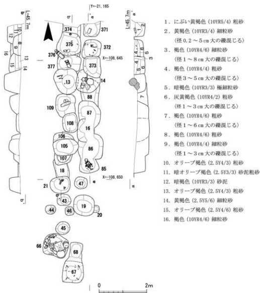
第72図 墓群 2 平面・断面図
