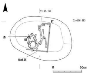
第102図 墓群14 S T 222・221・207・201・202・189実測図
