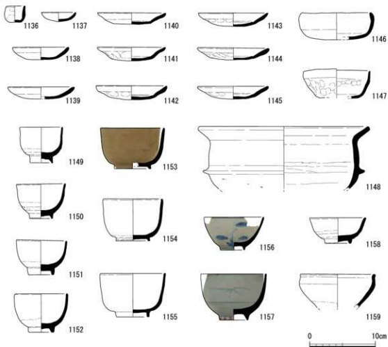
第137図 南地区墓地出土遺物実測図(20)
