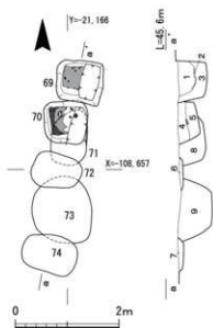
第90図 墓群11 平面・断面図
