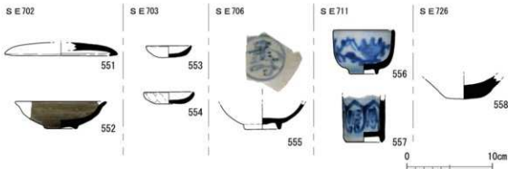
第62図 南地区出土遺物実測図(15)
