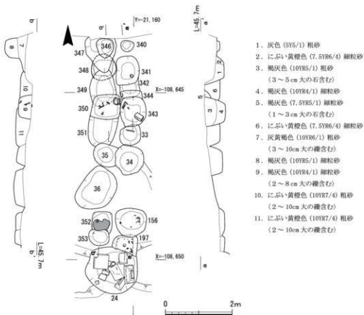
第76図 墓群4 平面・断面図
