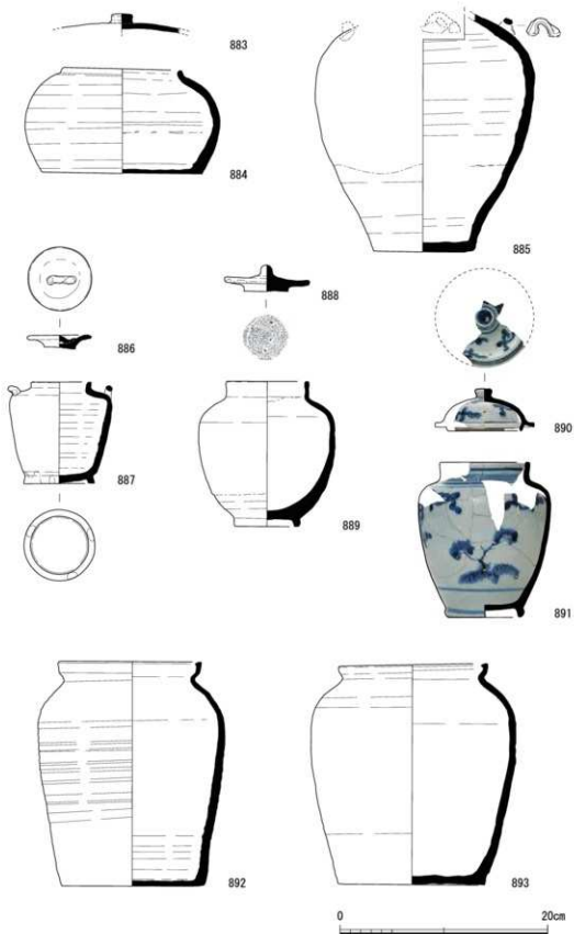
第127図 南地区墓地出土遺物実測図(10)
