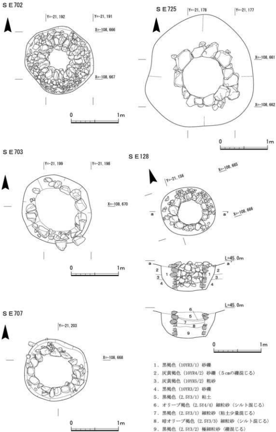
第44図 南地区遺構実測図(6)
