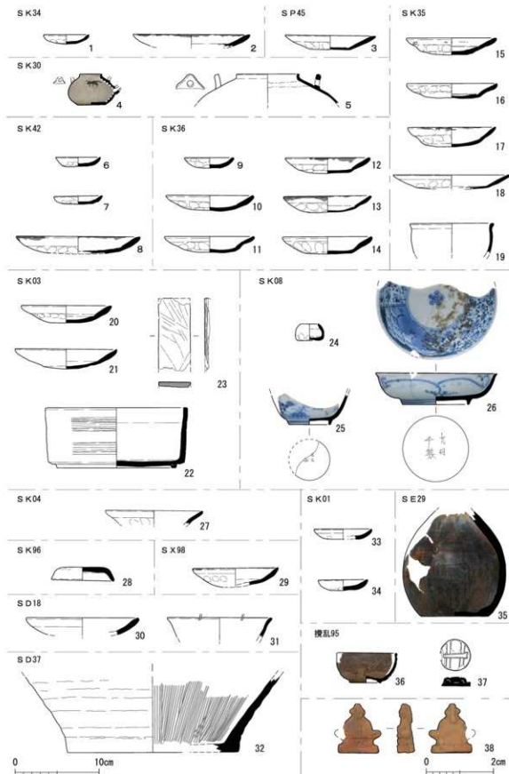
第21図 北地区出土遺物実測図(1)
