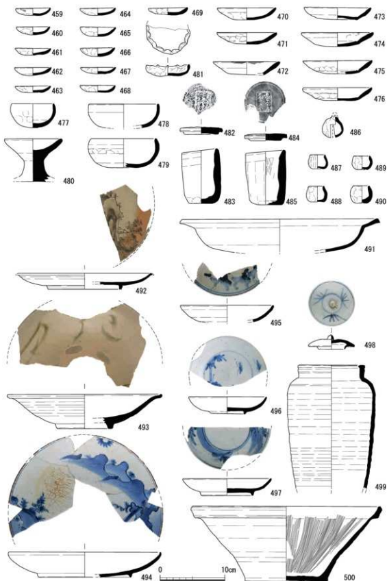
第59図 南地区出土遺物実測図(12)
