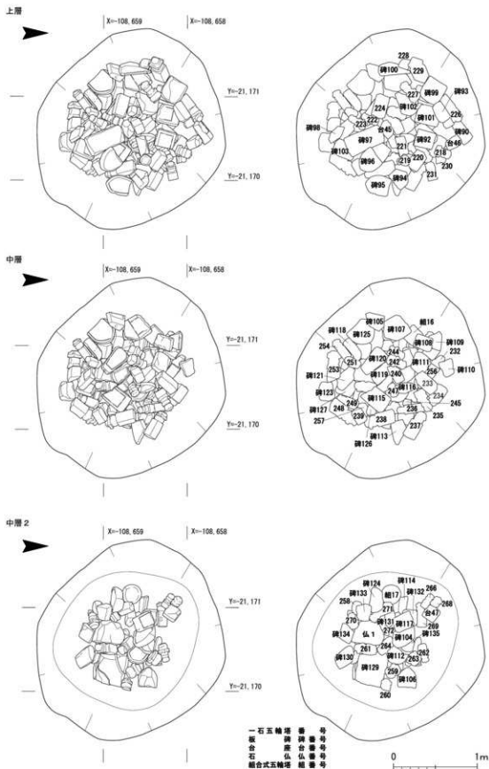
第114図 南地区SE113実測図(1)
