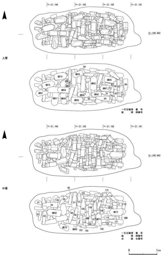
第111図 南地区S K 99実測図(1)
