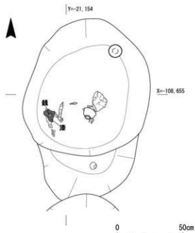
第97図 墓群13 S T127・415・416・230実測図
