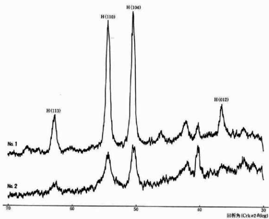
第13図 X線回折図(H:赤鉄鉱)
