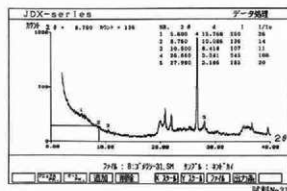
第 8 図 X線回折チャート(4)
