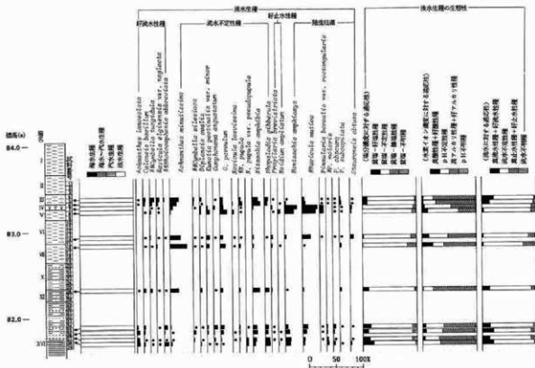
淡水・汽水・淡水生産産出率・各種産出率は全体基数、淡水生種の生態性の比率は淡水生産の合計を基数として算出した。いずれも100個体以上検出された試料について示した。なお、●は1%未満の産出を示す。
