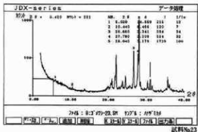
第7図 X線回折チャート(3)
