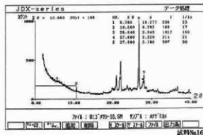
第6図 X線回折チャート(2)
