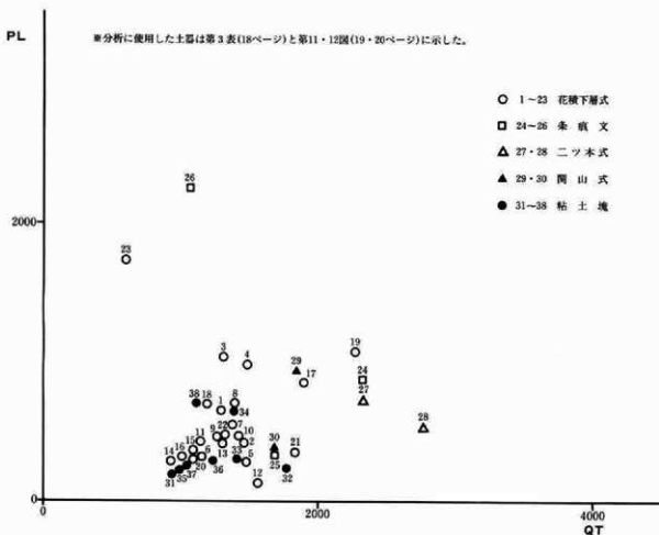
第4図 QT-PL 相関図
