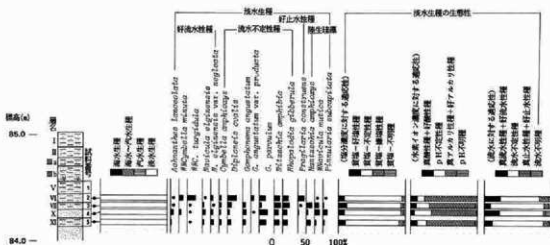
海水-汽水-淡水性種産出率・各種産出率は全体基数、淡水性種の生態性の比率は淡水性種の合計を基数として算出した。いずれも100個体以上検出された試料について示した。なお、●は1%未満の産出を示す。
