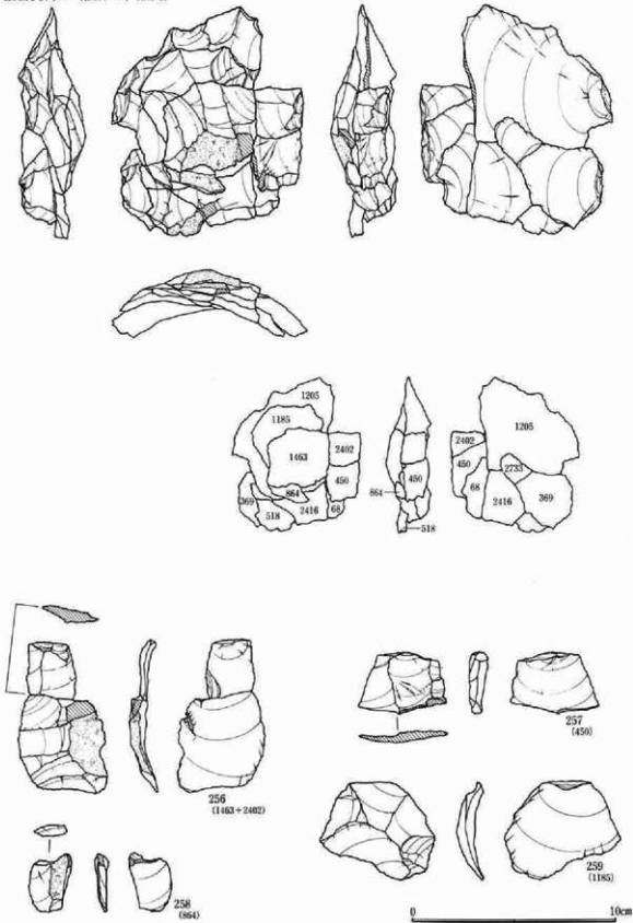
第57図 第I文 接合・個体別資料
