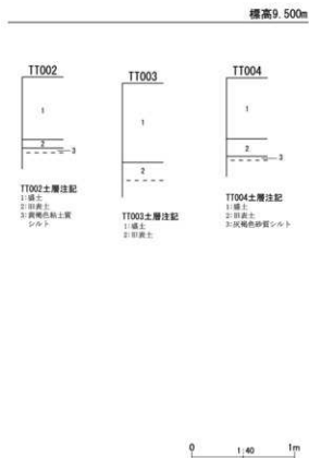
第 15 図 整理番号 20-2-305 試掘調査実施箇所及び土層断面模式図
