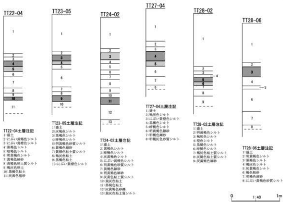
第29図 整理番号 20-2-313 試掘調査実施箇所及び土層断面模式図
