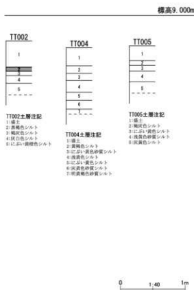
第33図 整理番号 20-2-318 試掘調査実施箇所及び土層断面模式図
