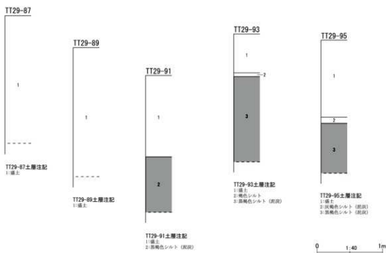
第 8 図 整理番号 15-3-322 試掘調査土層断面模式図
