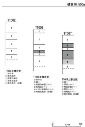
第14図 整理番号 20-2-301 試掘調査実施箇所及び土層断面模式図
