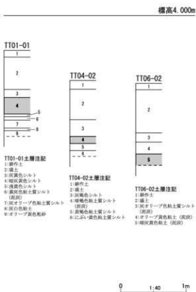
第 31 図 整理番号 20-2-315 試掘調査実施箇所及び土層断面模式図
