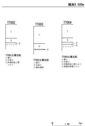
第 19 図 整理番号 20-2-308 試掘調査実施箇所及び土層断面模式図
