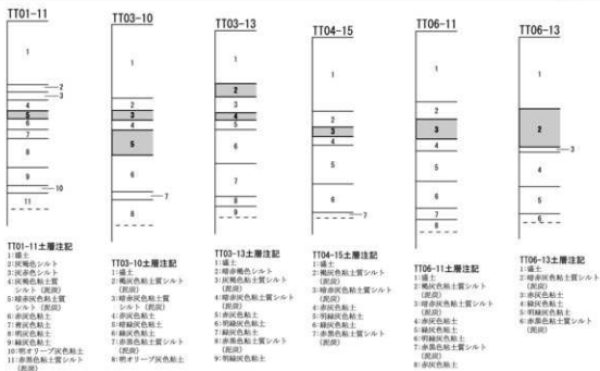
第11図 整理番号 20-3-306 試験調査実施箇所及び土層断面模式図
