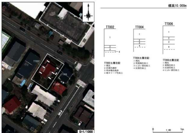
第 28 図 整理番号 20-2-311 試掘調査実施箇所及び土層断面模式図
