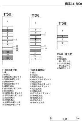
第13図 整理番号 19-2-315 試掘調査実施箇所及び土層断面模式図
