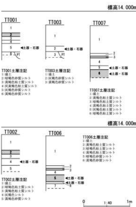
第21図 整理番号 20-2-310 試掘調査実施箇所及び土層断面模式図
