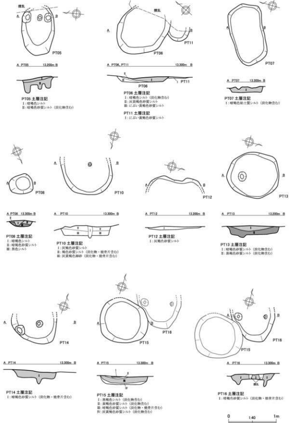
第24図 整理番号20-2-310 土坑実測図(2)
