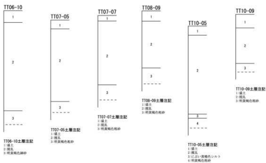
第 10 図 整理番号 20-3-305 試掘調査実施箇所及び土層断面模式図
