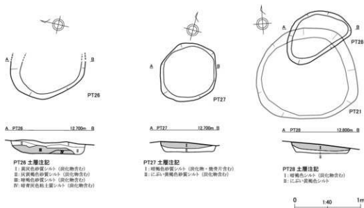
第26図 整理番号20-2-310 土坑実測図(4)
