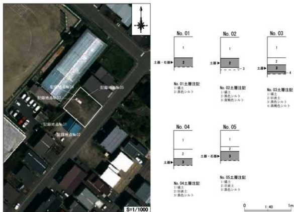
第34図 整理番号 19-2-313 工事立会実施箇所及び土層断面模式図
