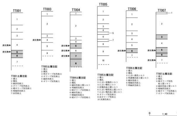
第9図 整理番号 19-3-314 試掘調査実施箇所及び土層断面模式図
