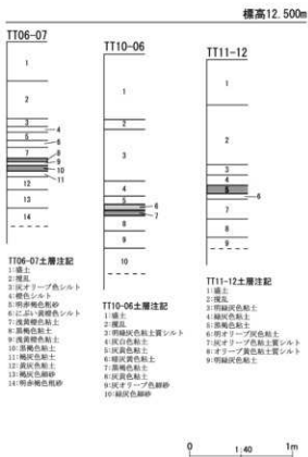
第 30 図 整理番号 20-2-314 試掘調査実施箇所及び土層断面模式図
