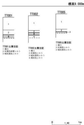
第32図 整理番号 20-2-317 試掘調査実施箇所及び土層断面模式図
