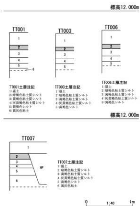
第 16 図 整理番号 20-2-306 試掘調査実施箇所及び土層断面模式図
