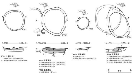
第 23 図 整理番号 20-2-310 土坑実測図 (1)
