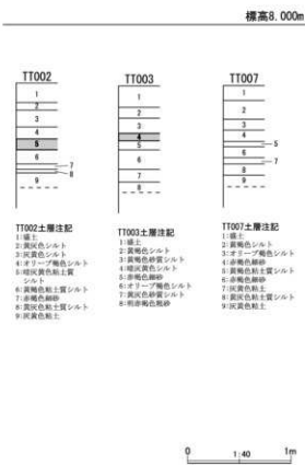
第20図 整理番号 20-2-309 試掘調査実施箇所及び土層断面模式図
