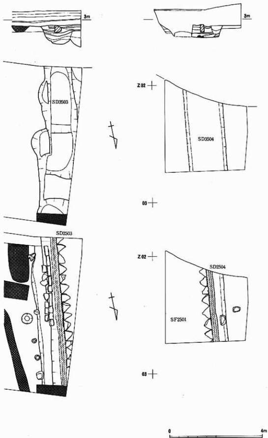
第34図 SF2501と側溝
