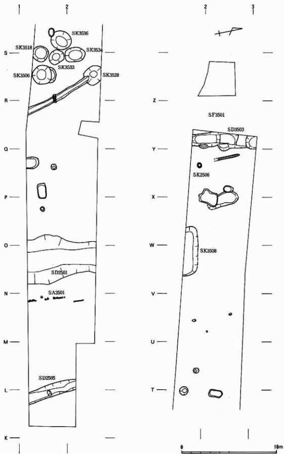
第52图 西中ノ町2・3区下層平面图
