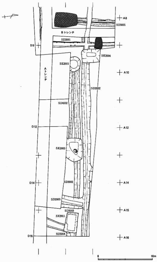
第16図 東中ノ町地区平面図(1)
