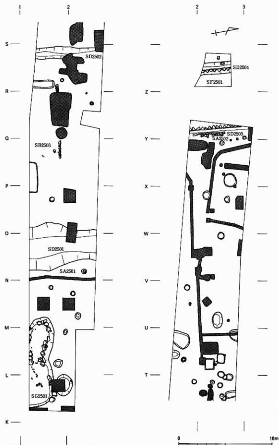
第31图 西中ノ町2・3区上層平面图
