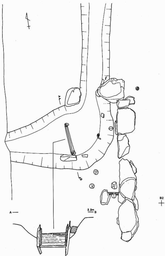
第40圖 SD2201と埴
