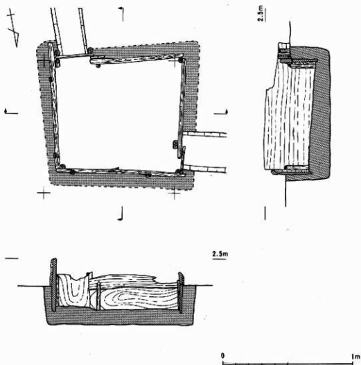
第38図 中ノ町B地区平面図(上層)と西壁断面図
