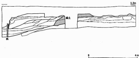
第14図 西外堀・土塁跡断面図
