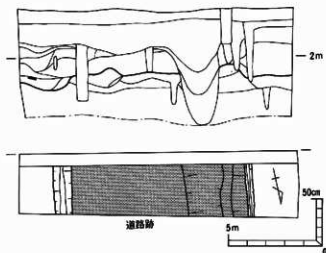
第10図 東中ノ町地区2トレンチ道路跡
