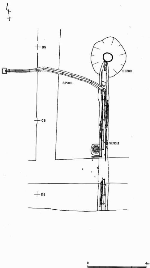
第27圖 SD3011とSP2001
