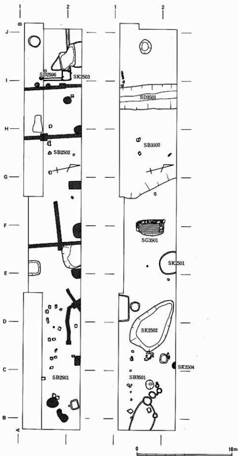
第48图 西中ノ町1区平面图(左:上层, 右:下层)
