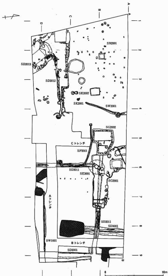
第17図 東中ノ町地区平面図(2)
