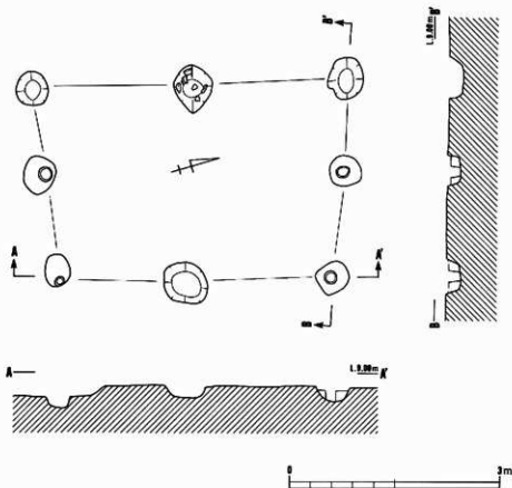
第115図 掘立柱建物 9
