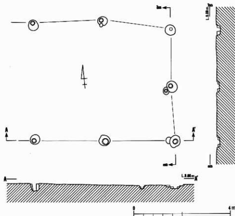
第114図 掘立柱建物 8
