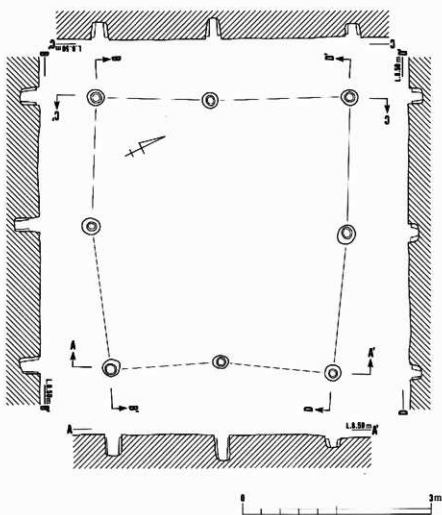
第112図 掘立柱建物6
