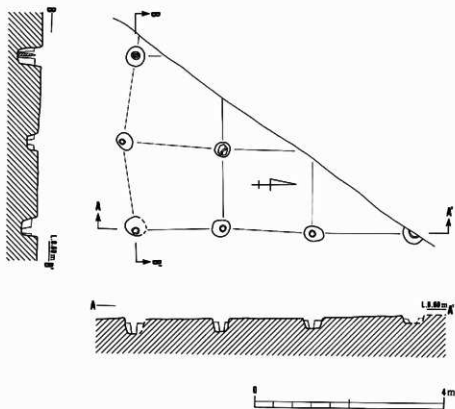
第122図 掘立柱建物10
