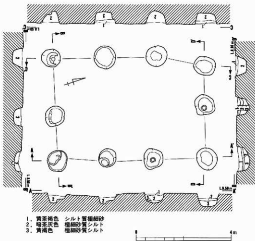
第113図 掘立柱建物 7
