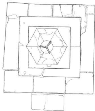
上蓋図
