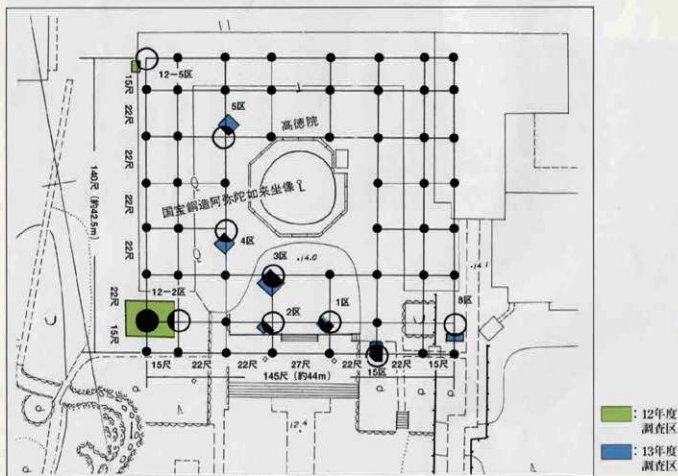
大仏殿の規模（推定図） Daibutsuden's scale (estimated figure).
