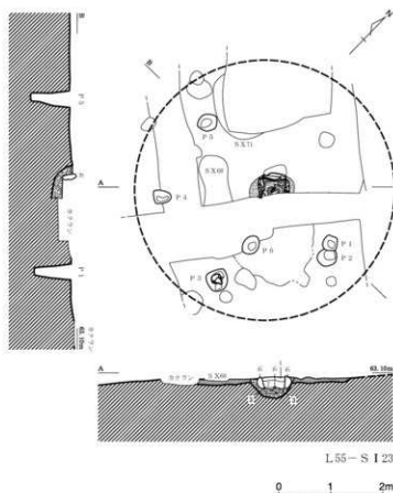
1. L.55-S I 23 実測図 (1/80)
