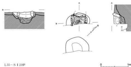
1. L.55-S I 23 実測図 (1/80)
