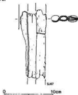
第89图 第21号方形周溝墓出土鉄製品、第41号方形周溝墓出土木製品、 第17・67号住居跡出土炭化材実測図
