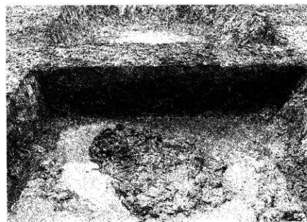
第12号方形周溝墓 南溝土層断面
