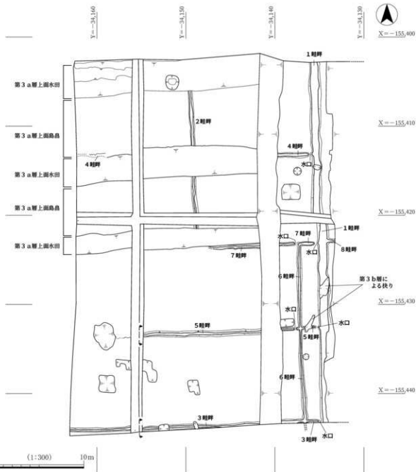
図11 第4a層上面 平面図
