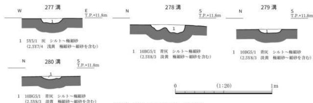
図 31 第 9 a 層上面 溝 断面図
