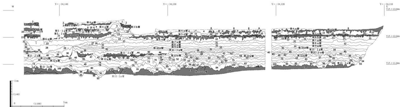
图7 1区 东西 (X=-155,420) 断面图
