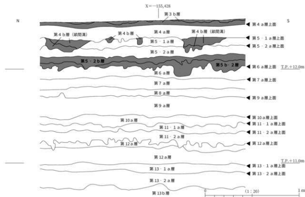
図5 基本層序（1区南北断面 図6の部分拡大）
