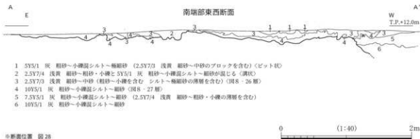
図29 第7 a層上面 79 溝東部遺構群 断面図
