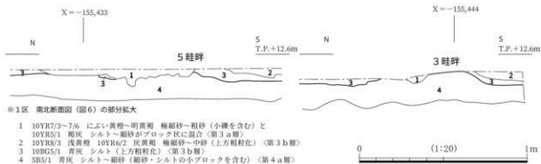
図12 第4a層上面 畦畔 断面図 (Y = - 34,155)
