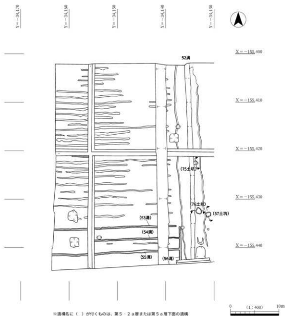
図16 第5-2 a層上面・下面 平面図
