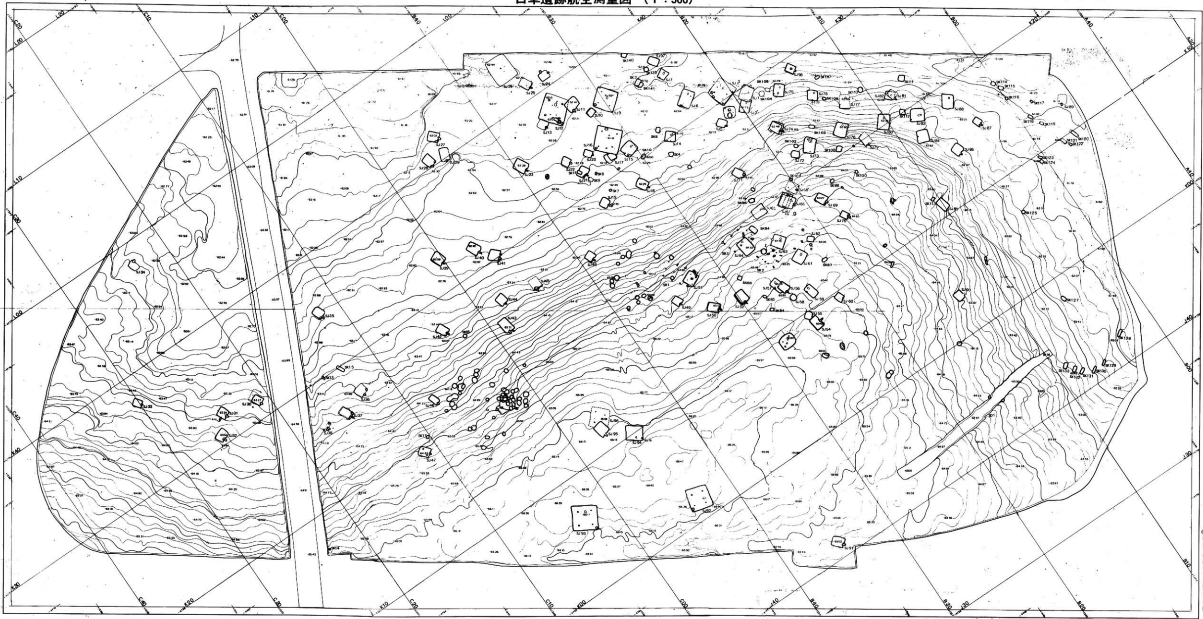
白草遺跡航空測量圖 (1:500)
