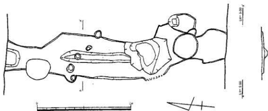
第10図 1号溝実測図 (1/100)
