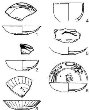
第7図 1号掘立柱建物出土遺物 (1/4)
