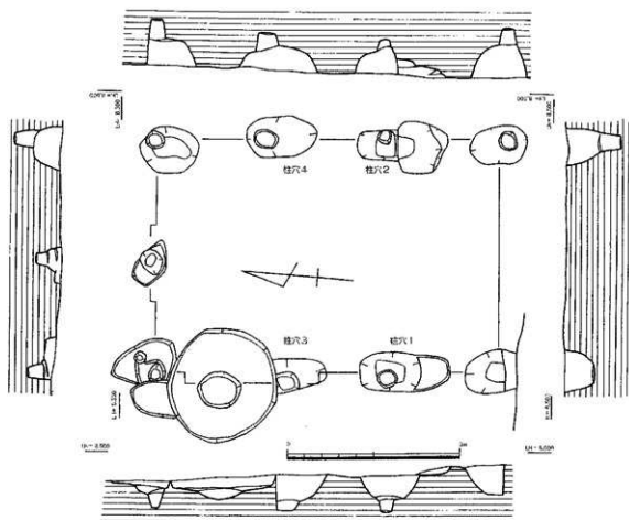
第6図 1号掘立柱建物実測図 (1/60)
