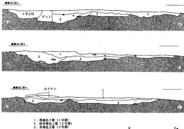
Fig. 3 溝状遺構土層断面図 (1/40)
