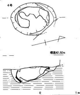
Fig. 8 3号·4号甕棺墓实测图(1/30)
