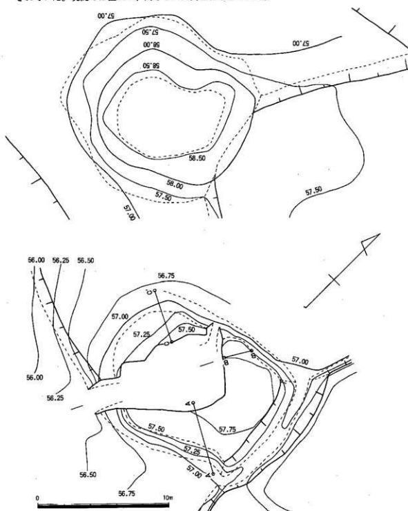
Fig. 34 3号墳現況・地山整形測量図(1/200)
