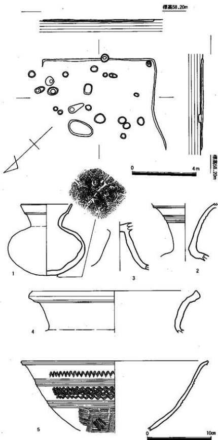
Fig. 38 住居跡・出土遺物実測図(1/60・1/3)
