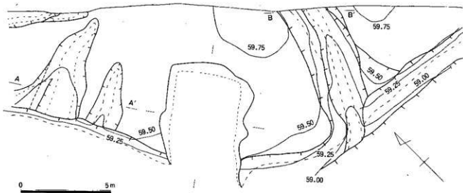
Fig.20 1号墳地山整形測量図(1/150)
