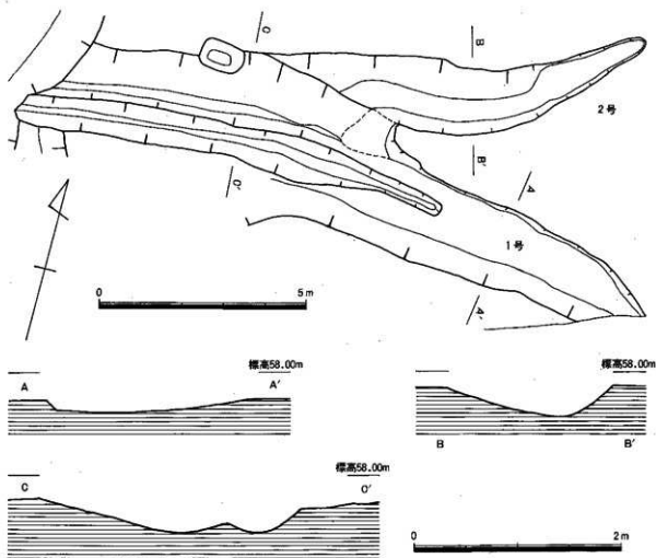
Fig. 40 1～2号溝・断面実測図(1/100・1/40)
