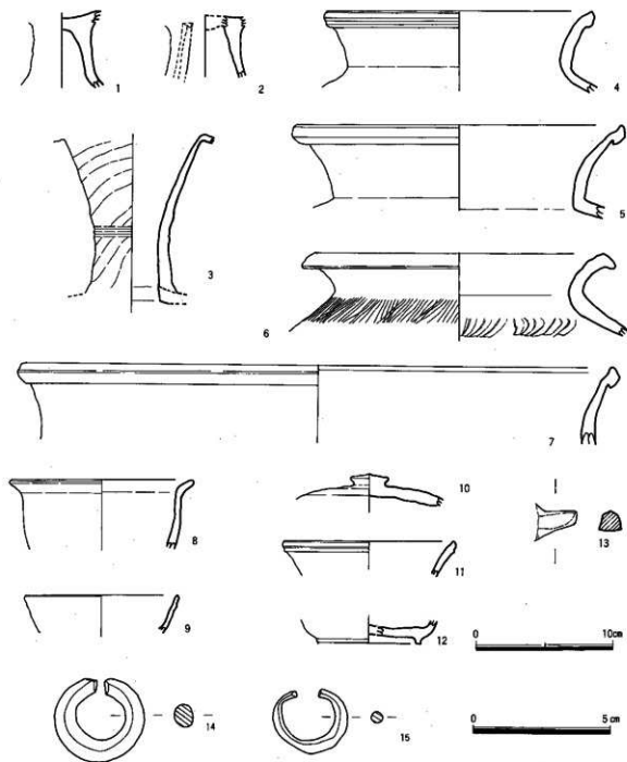
Fig.22 出土遺物実測図(1/3・2/3)
