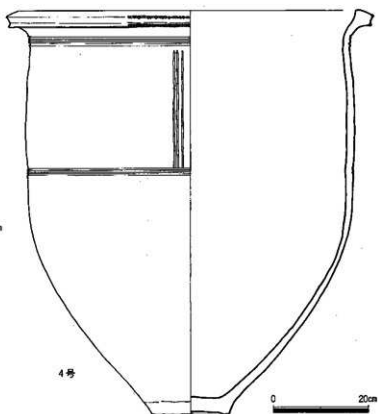
Fig. 9 3号·4号甕棺墓实测图(1/8)
