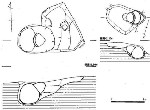
Fig.13 7号・8号変棺墓実測図(1/30)
