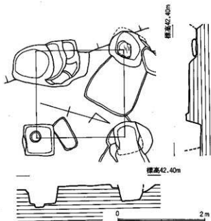
Fig.18 掘立柱建物実測図(1/60)
