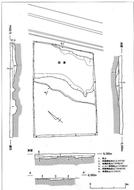
図17. 御願塚古墳第5次調査実測図
