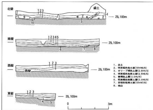
図9. 伊丹廃寺跡第37次調査実測図
