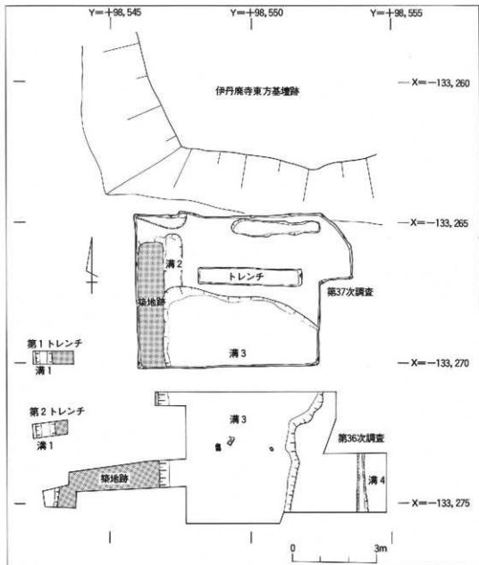
図19. 伊丹廃寺跡第36次・第37次調査実測図
