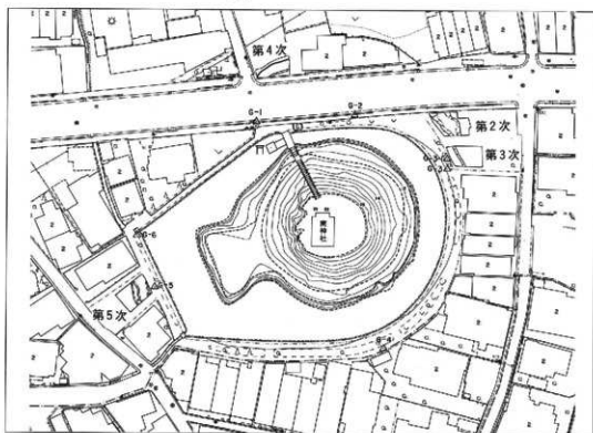
図20. 御願塚古墳実測図(1/1,000)
