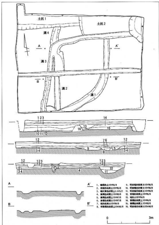
図13. 緑ヶ丘遺跡第5次調査A地区実測図
