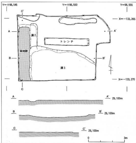
図8. 伊丹廃寺跡第37次調査実測図
