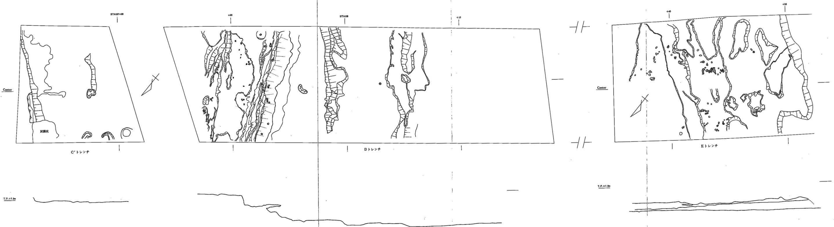
付図5 C'・D・Eトレンチ中世長瀬川河床面平面図・断面図 (1/500)
