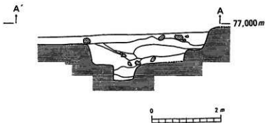
第5図 墾地跡実測図
