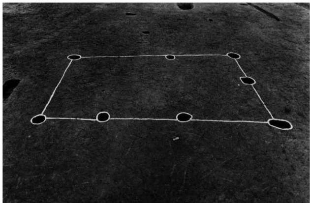
第28号掘立柱建物跡
