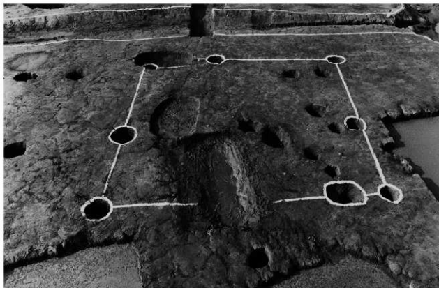
第30号掘立柱建物跡
