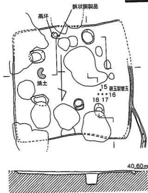
第37図 1・2号住居実測図 (1/60)
