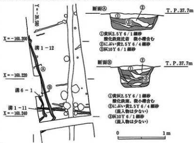
第12図 溝1-11・12 溝6-1平面図(1000分の1) 断面図(40分の1)
