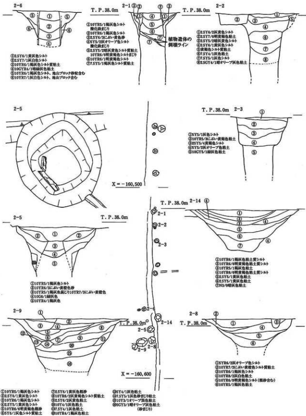
第87図 近世井戸(3) 平面図・断面図(80分の1)
