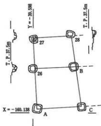
第24図 掘立柱建物1-3平面図・断面図(100分の1)
