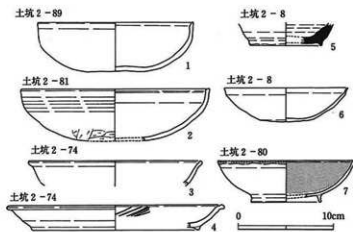
第76図 土坑出土遺物（4分の1）
