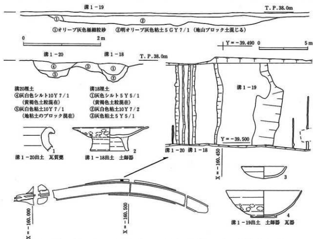
第79図 陌線V 溝1-18・19・20平面図(200分の1)・断面図(40分の1)・出土遺物(4分の1)
