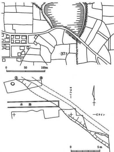
第51図 溝3-2位置図(3000分の1)・平面図(200分の1)
