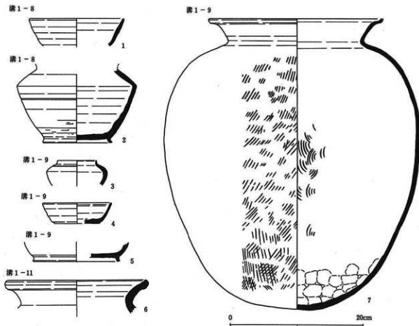
第14図 溝1-8・9・11出土遺物(4分の1)
