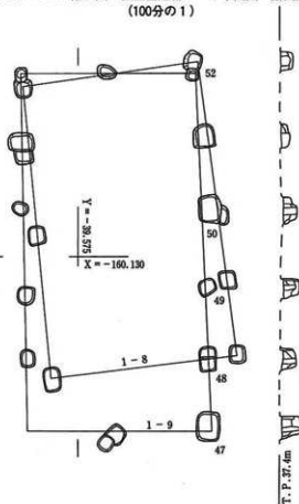
第25図 掘立柱建物1-8・9平面図・断面図(100分の1)
