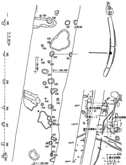
第38図 構2-1平面図・断面図(100分の1)
