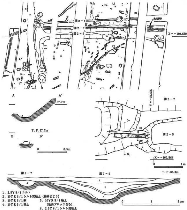
第80図 陌線Ⅵ 坪境溝2-5・6・7平面図・断面図(500分の1) 溝2-5木樋平面図(40分の1)・同断面図(20分の1) 出土遺物(4分の1)
