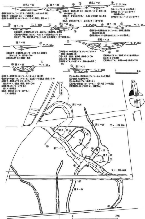
第11圖 溝 7-23・24・25・26・65 土坑 7-33平面圖 (200分の1) 断面圖 (40分の1)
