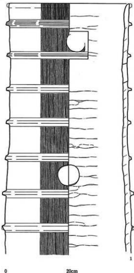
第17図 棺転用円筒埴輪 (6分の1)
