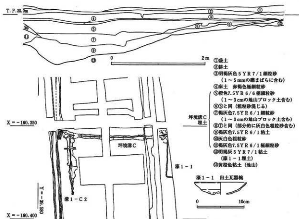
第78図 陌線Ⅳ 坪境溝平面図(1000分の1)・断面図(40分の1)
