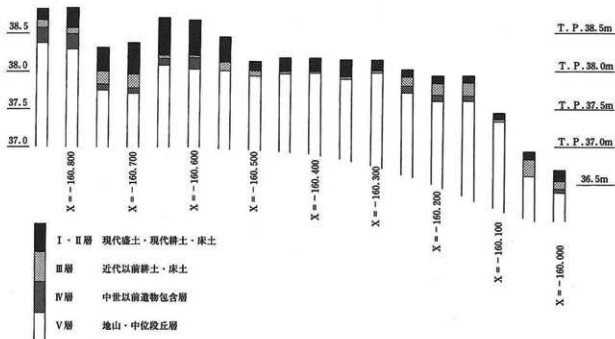
第6図 土層断面模式図
