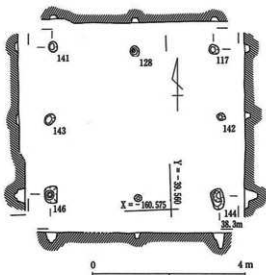
第57図 掘立柱建物 2-3 平面図・断面図 (100分の1)
