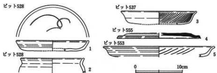
第39図 構2-1ピット出土遺物(4分の1)
