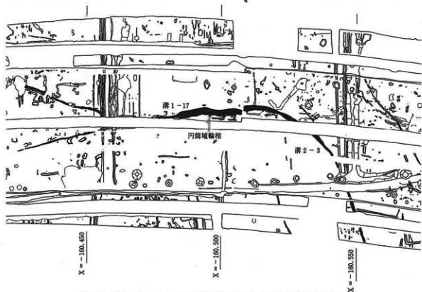
第15図 溝1-17・2-3平面図(1000分の1) 出土遺物(4分の1)
