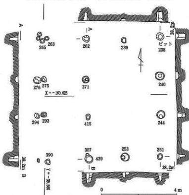
第67図 掘立柱建物 2-7 平面図・断面図 (100分の 1)
