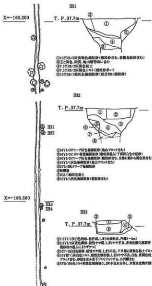
第88図 近世井戸(4)断面図(80分の1)
