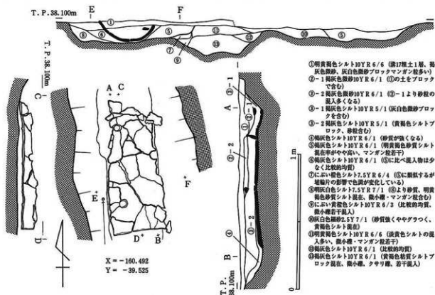
第16図 円筒埴輪筒棺平面図・断面図(20分の1)
