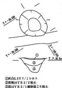
第75図 井戸2-19平面図・断面図 (40分の1)
