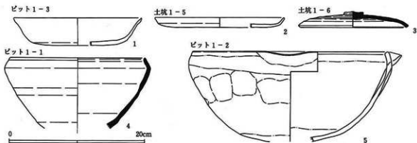
第32図 ビット・土坑出土遺物(4分の1)
