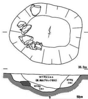
第62図 土坑 2-45平面図・断面図 (20分の1)
