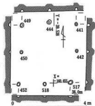
第70図 掘立柱建物 2-11平面図・断面図 (100分の1)
