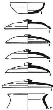
第10図 溝7-23出土遺物 (4分の1)
