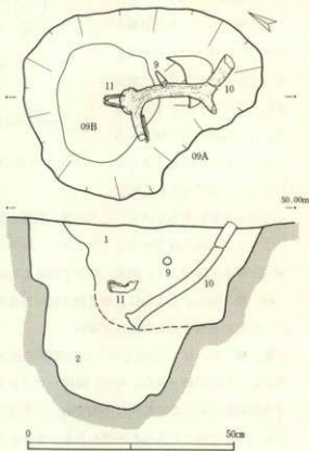
第9図 3T-09 (1:10)
