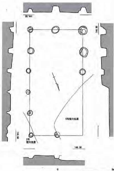
第33図 6号掘立柱建物実測図 (1/100)
