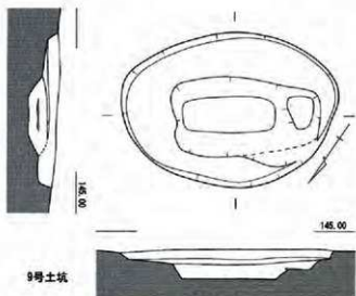
第38图 3~9号土坑实测图 (1/50)
