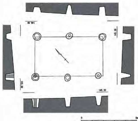
第29図 1号掘立柱建物実測図(1/100)
