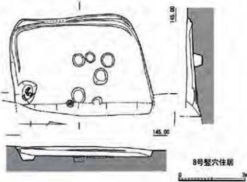
第10図 6～8号竪穴住居実測図（1/80）
