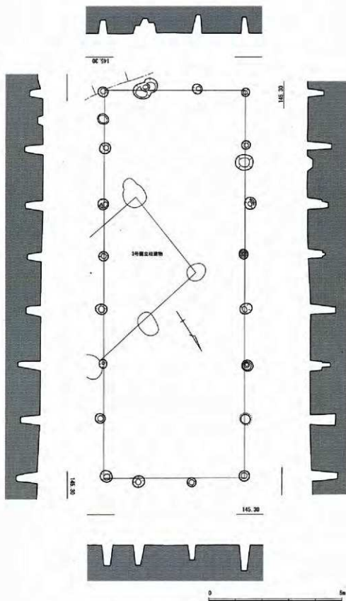
第 32 图 5 号掘立柱建物实测图 (1/100)
