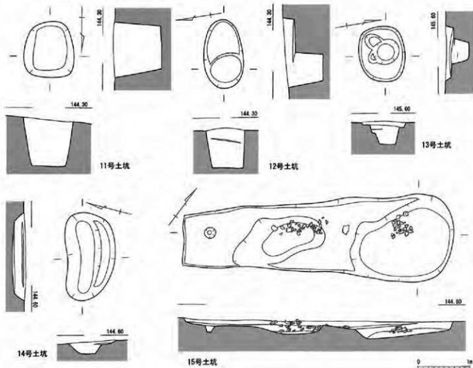
第39図 11～15号土坑実測図 (1/50)
