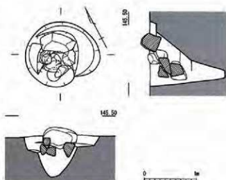
第22図 20号竪穴住居内ピット実測図（1/50）
