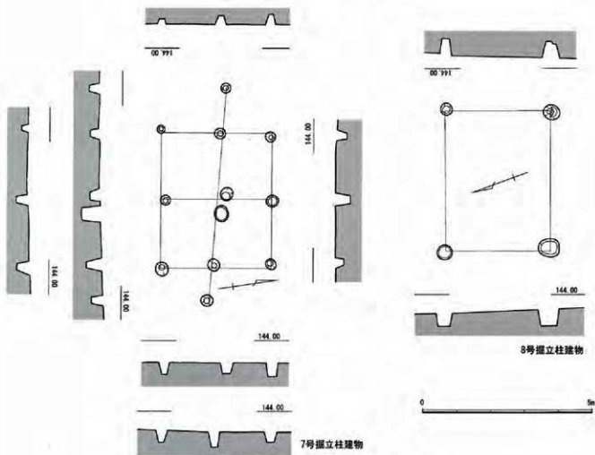
第34図 7・8号掘立柱建物実測図 (1/100)
