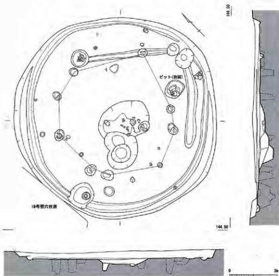
第21図 20号竪穴住居実測図(1/80)
