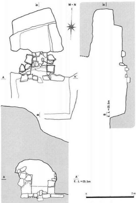
第4图 1号墓实测图
